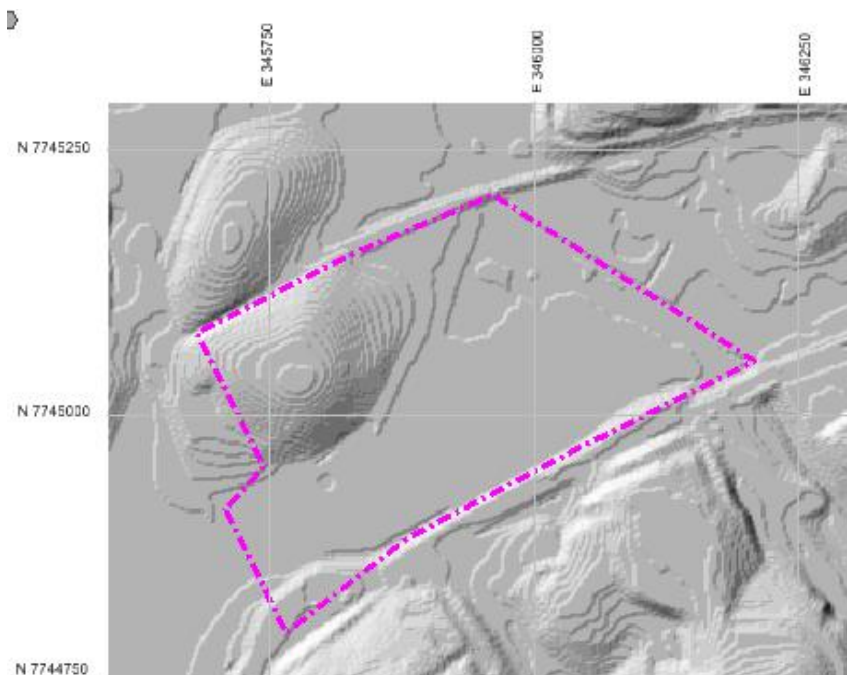
Figura 90: Modelo Digital de Terreno - MDT
