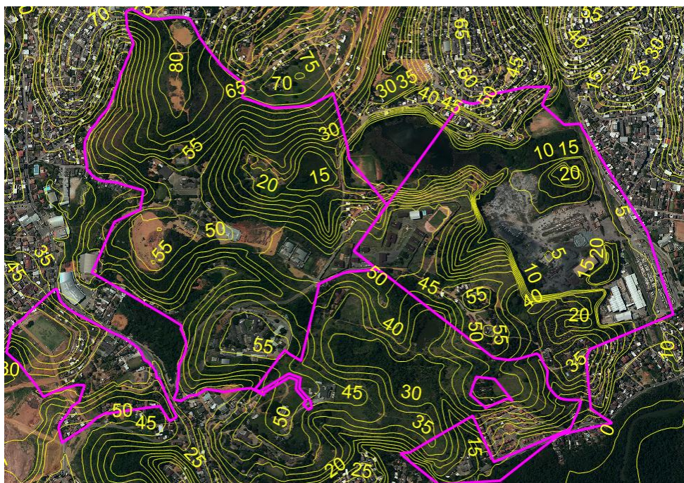
Figura 25: Curvas de nível
